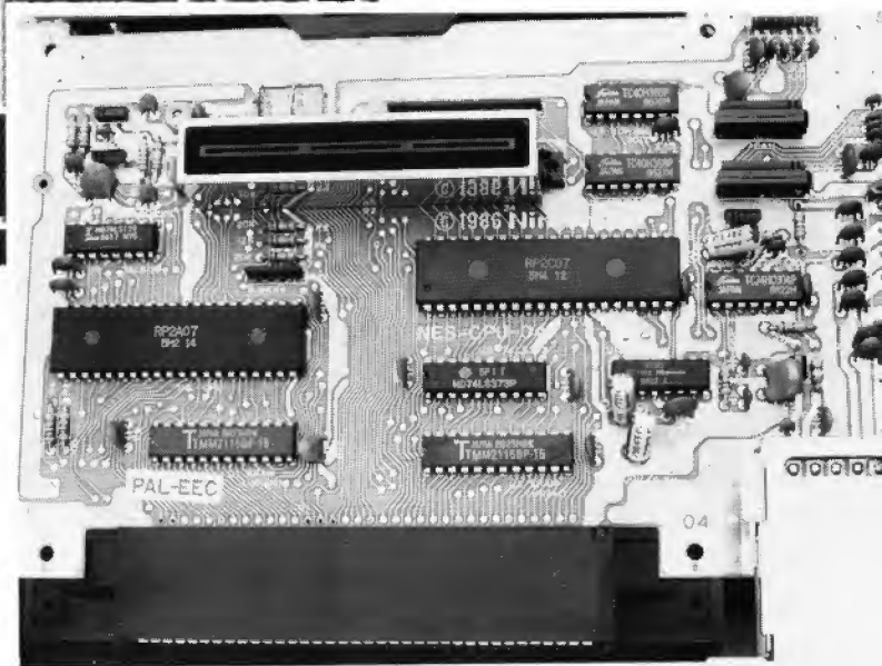
Sådan er Nintendoen ud indven-dig. Bemærk LSI-kredsene.
